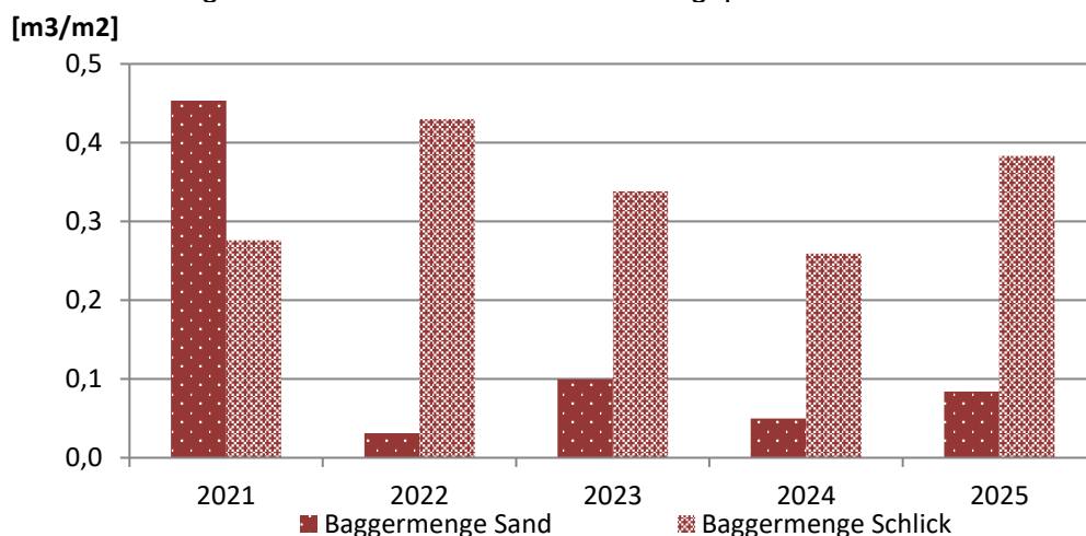
Abbildung 29: Baggermengen in den abgeschleusten Arealen Überseehafen und Fischereihafen (Schlick) und an der Strom- und Columbuskaje (Sand)
