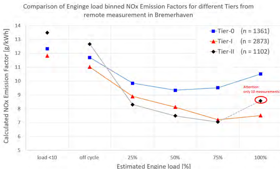
Abbildung 23: Vergleich der lastabhängigen NOx-Emissionsfaktoren für TIER-Normen 0, I und II an der BSH-Messstation Bremerhaven (Quelle: eigene Berechnung BSH)
