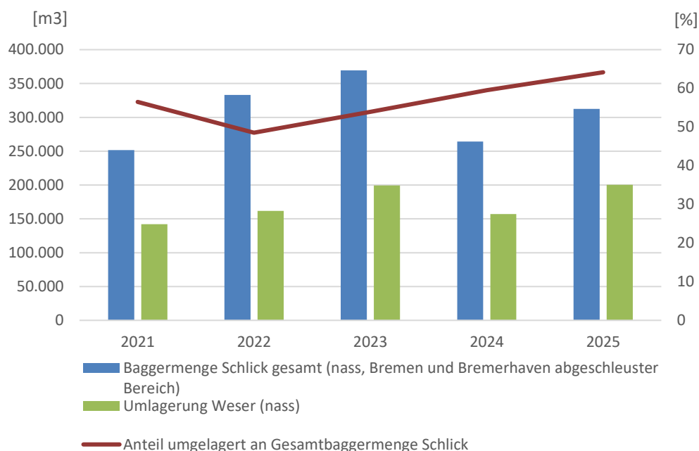
Abbildung 30: Mengen und Anteil der Umlagerung von schlickigem Baggergut in der Weser
