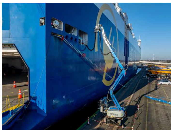
Abbildung 24: Landstromversorgung eines Autocarriers
