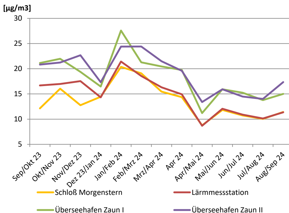
Abbildung 26: Stickstoffdioxidkonzentrationen an den verschiedenen Messorten
