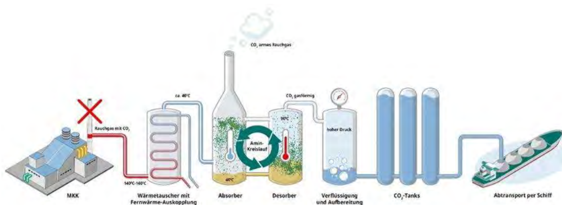
Abbildung 15: Schematische Darstellung des Abscheideprozesses Foto:swb
